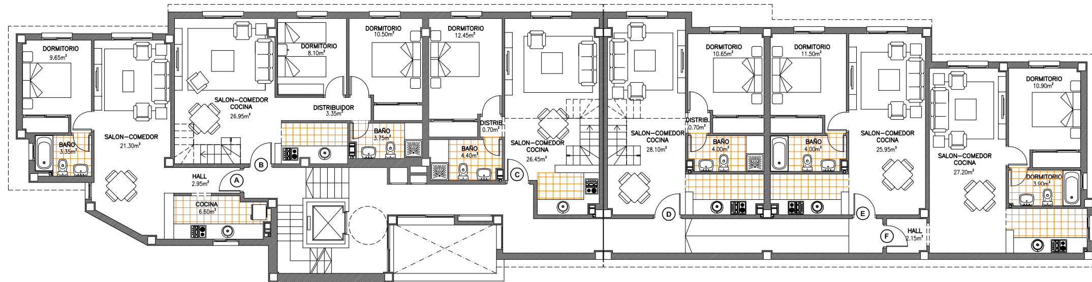
PLANTA SEGUNDA BLOQUE - 2
