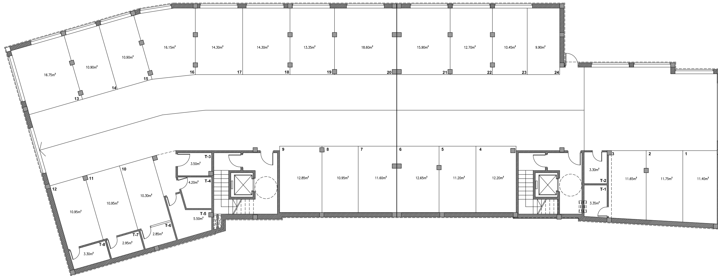
PLANTA SOTANO BLOQUE - 1
